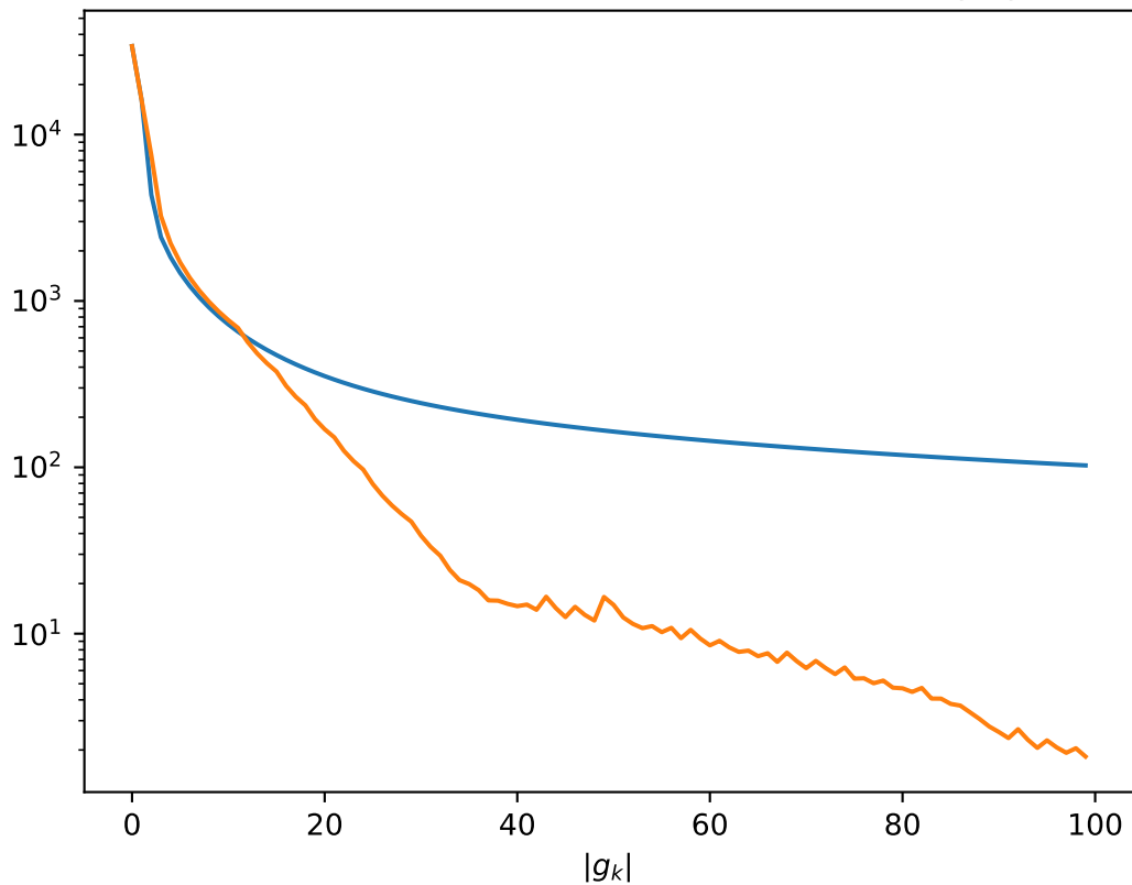
Gráfica de los métodos, iteraciones (k) vs. |g_k|
